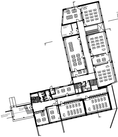
Grundriss EG
