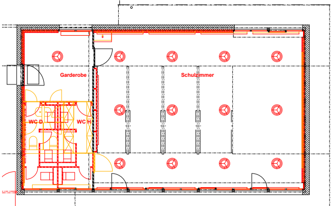
Grundriss Pavillon E 1:200
