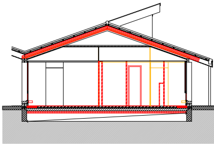
Querschnitt Pavillon E 1:200
