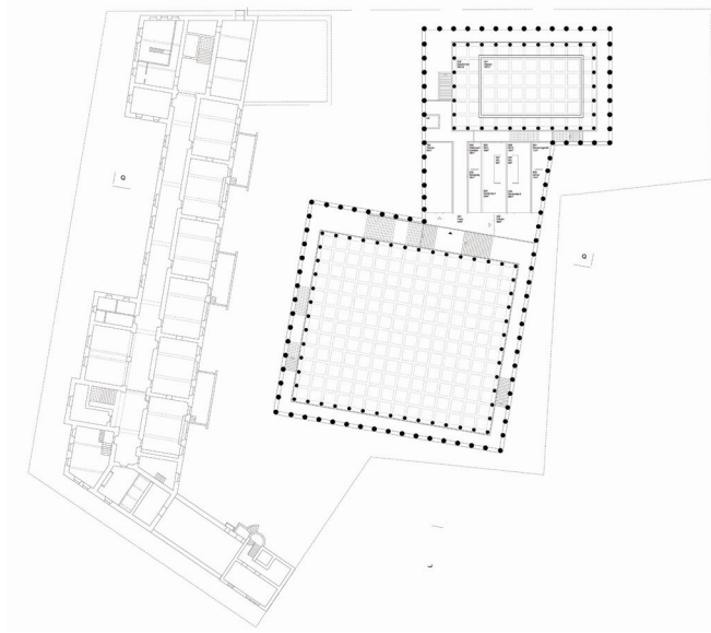
Grundriss 1. UG
