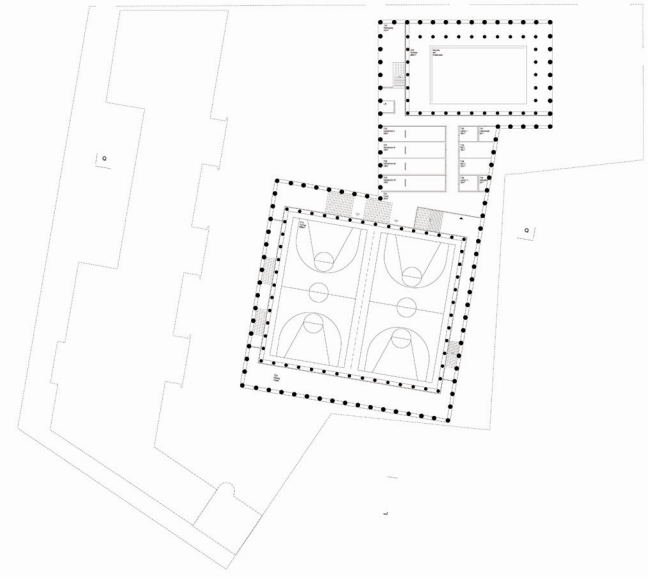
Grundriss 2. UG
