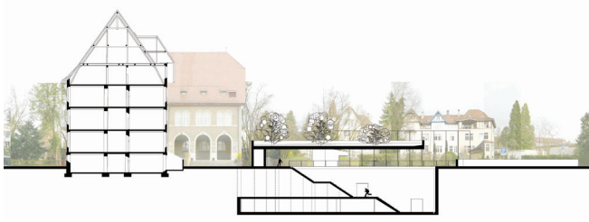
Querschnitt
