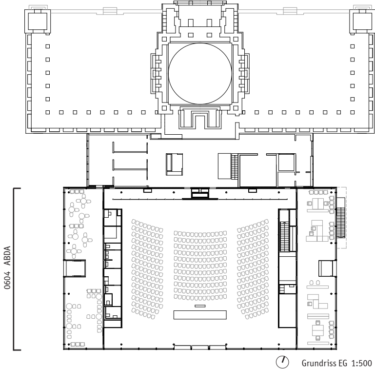
Grundriss EG 1:500
