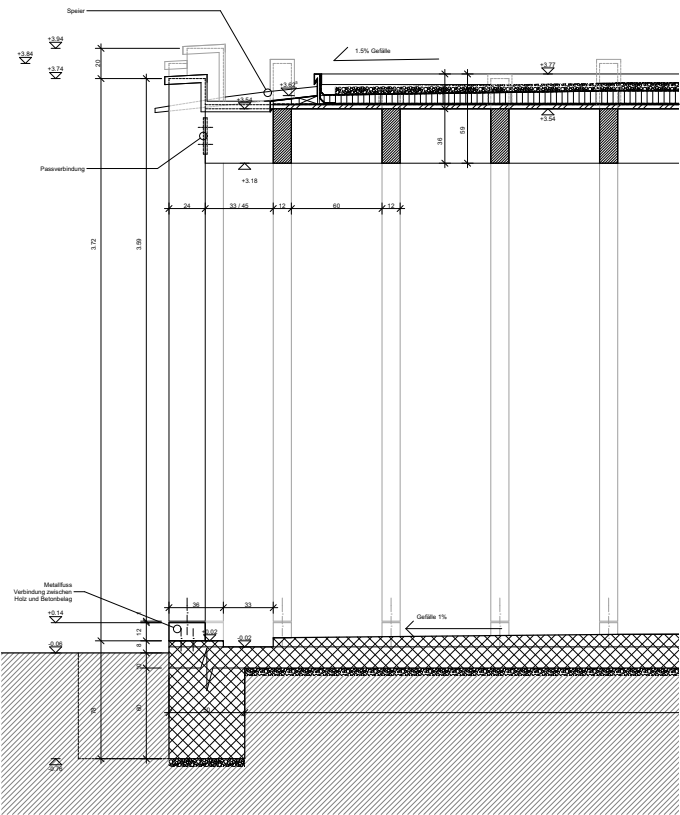
Detailschnitt 1:50
