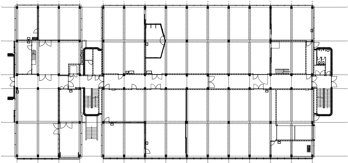
Grundriss Erdgeschoss 1:500
