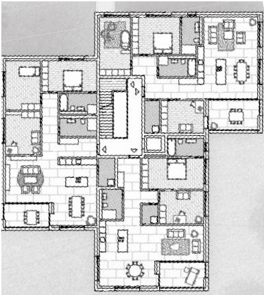
Typischer Grundriss 1:500
