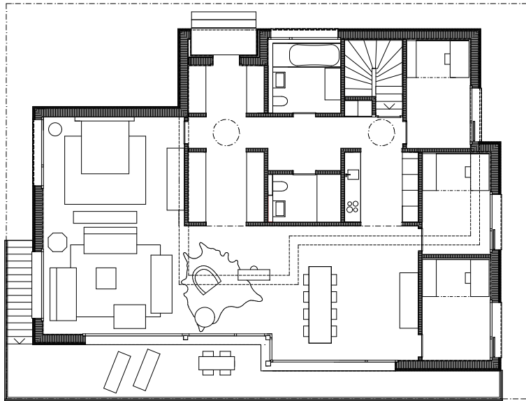
Grundriss Erdgeschoss 1:200
