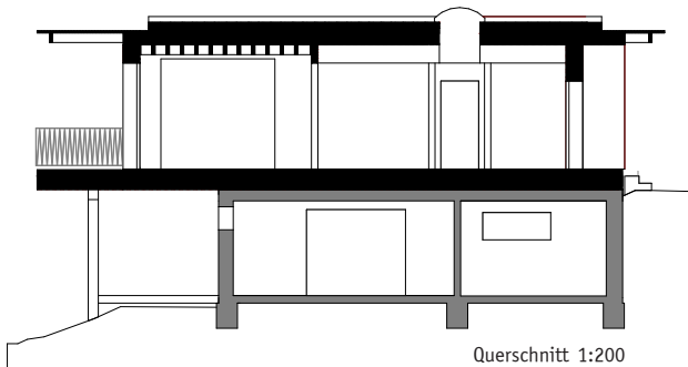
Querschnitt 1:200
