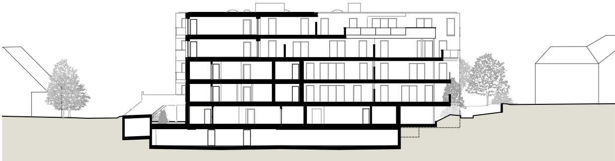
Längsschnitt 1:500
